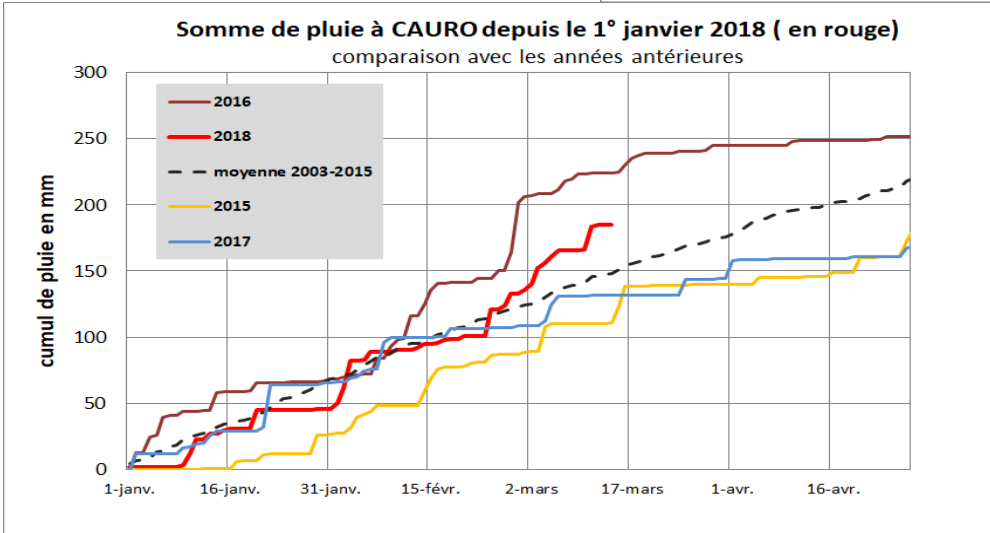
Graphique 3 : Cumul des précipitations à Cauro
